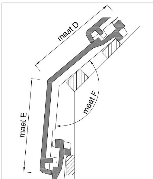
mansarde knikpan op maat
