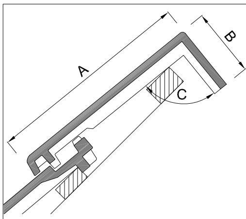
Chaperonpan op maat
