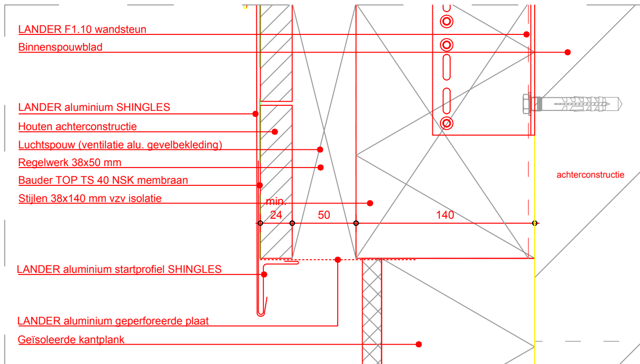
Maaiveld aansluitdetail V-01
