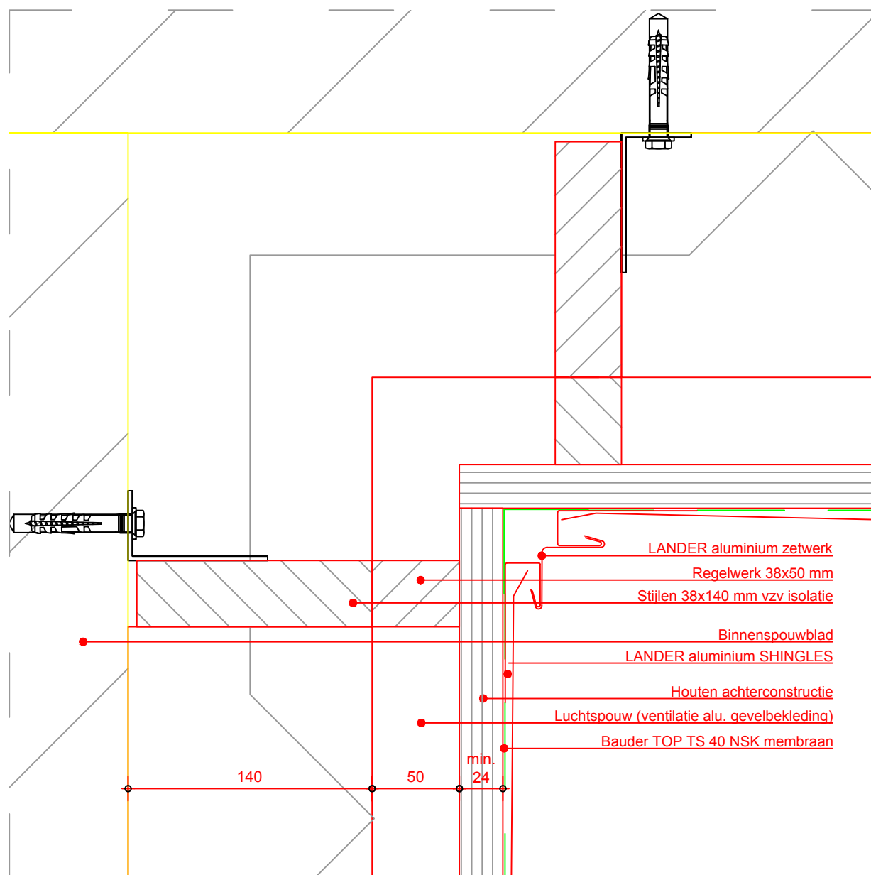
Binnenhoekdetail H-02a
