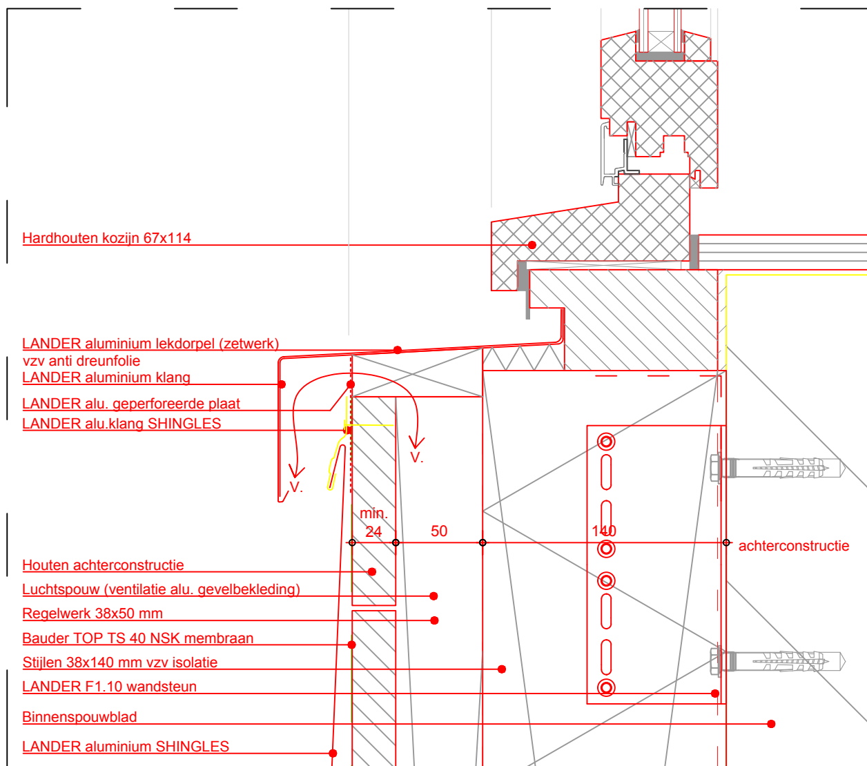
Aansluitdetail onderdorpel V-04
