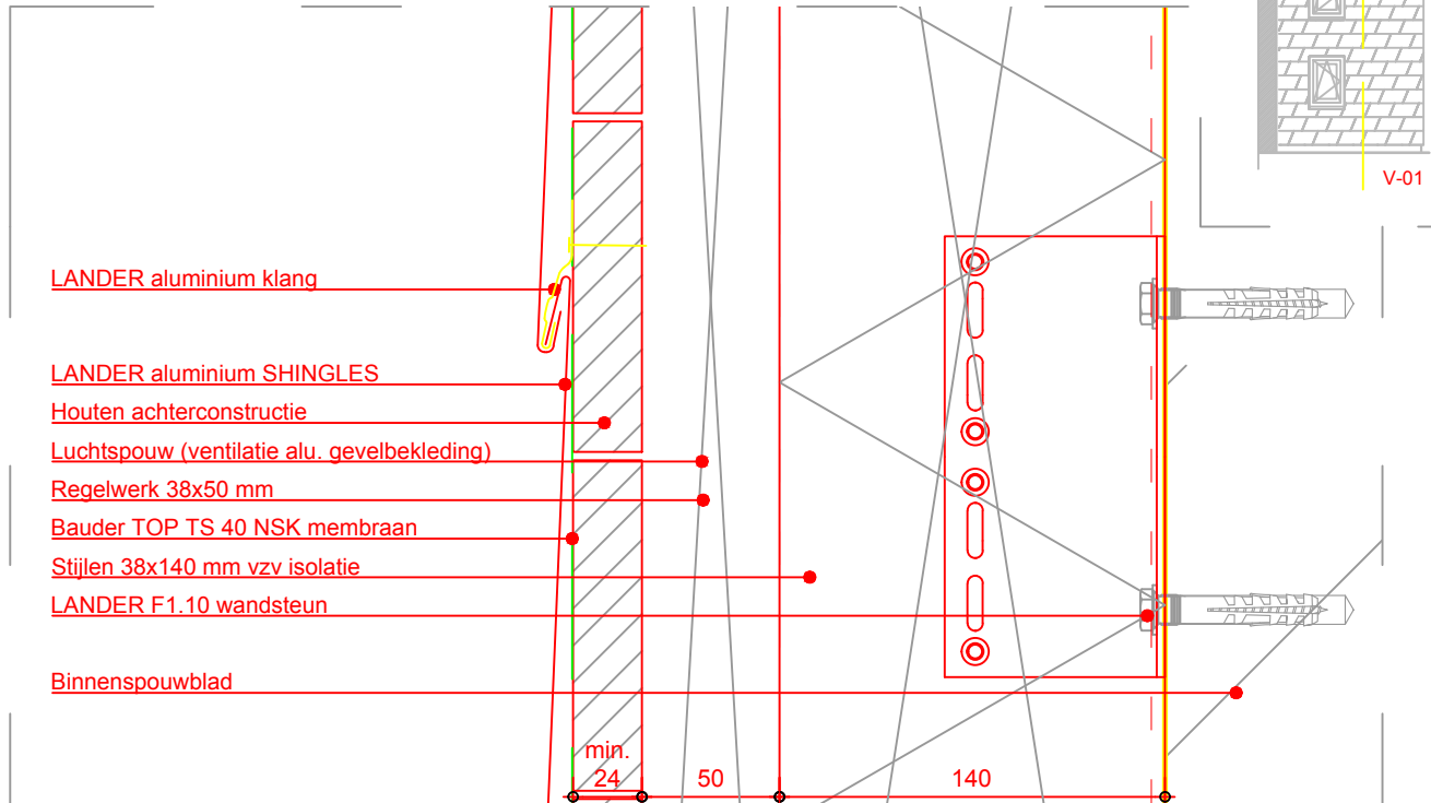
Aansluitdetail SHINGLES V-02
