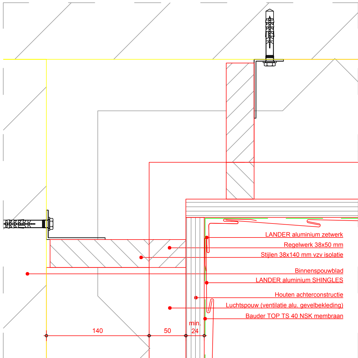
Binnenhoekdetail H-02a
