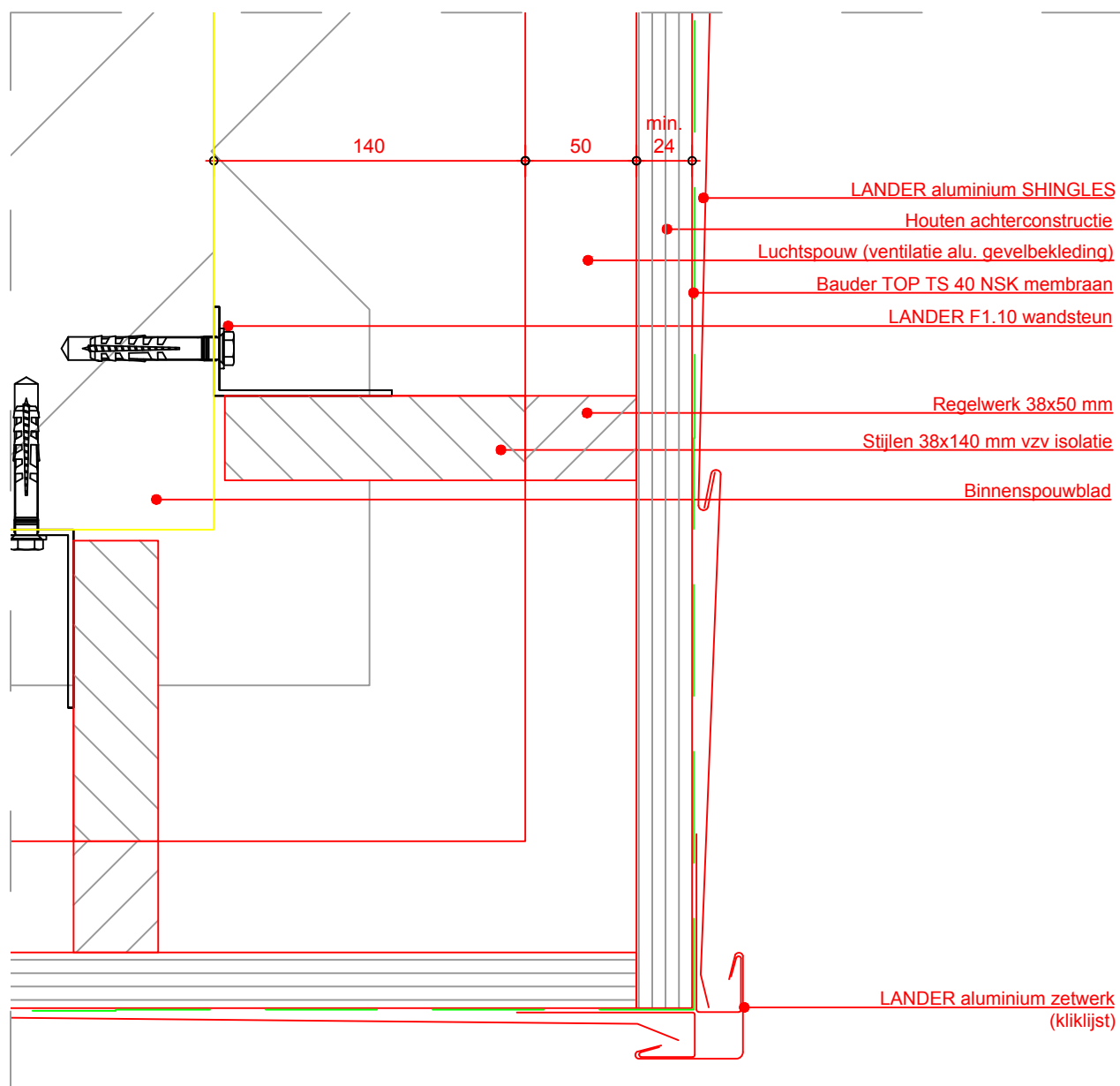
Buitenhoekdetail H-01b
