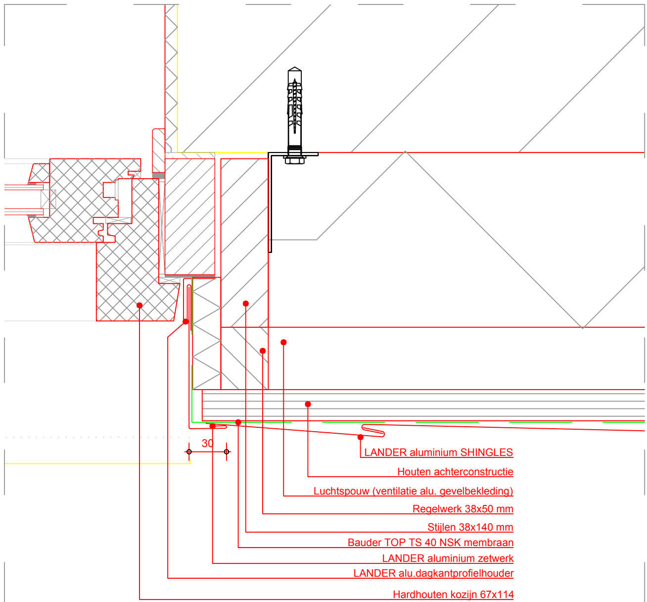
Aansluitdetail kozijnstijl H-03a
