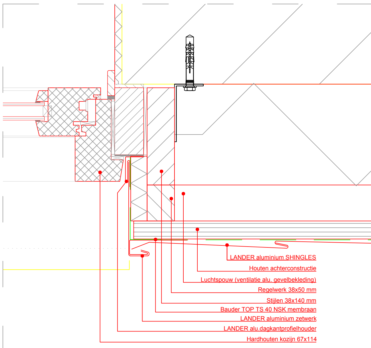
Aansluitdetail kozijnstijl H-03b
