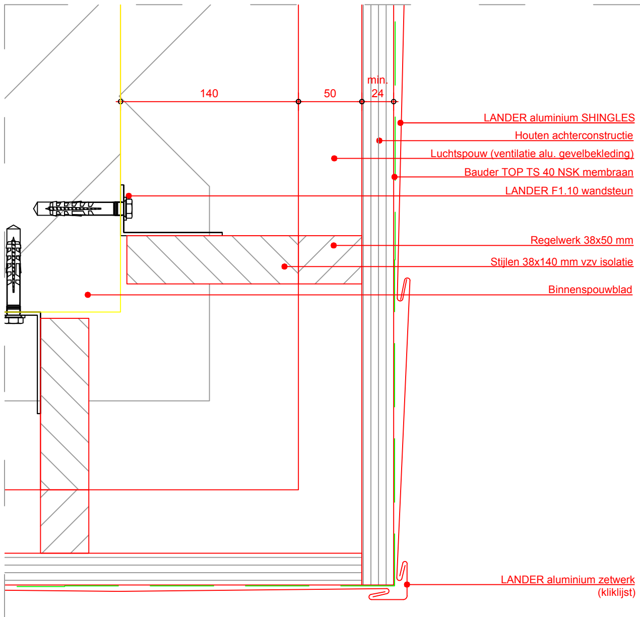
Buitenhoekdetail H-01c
