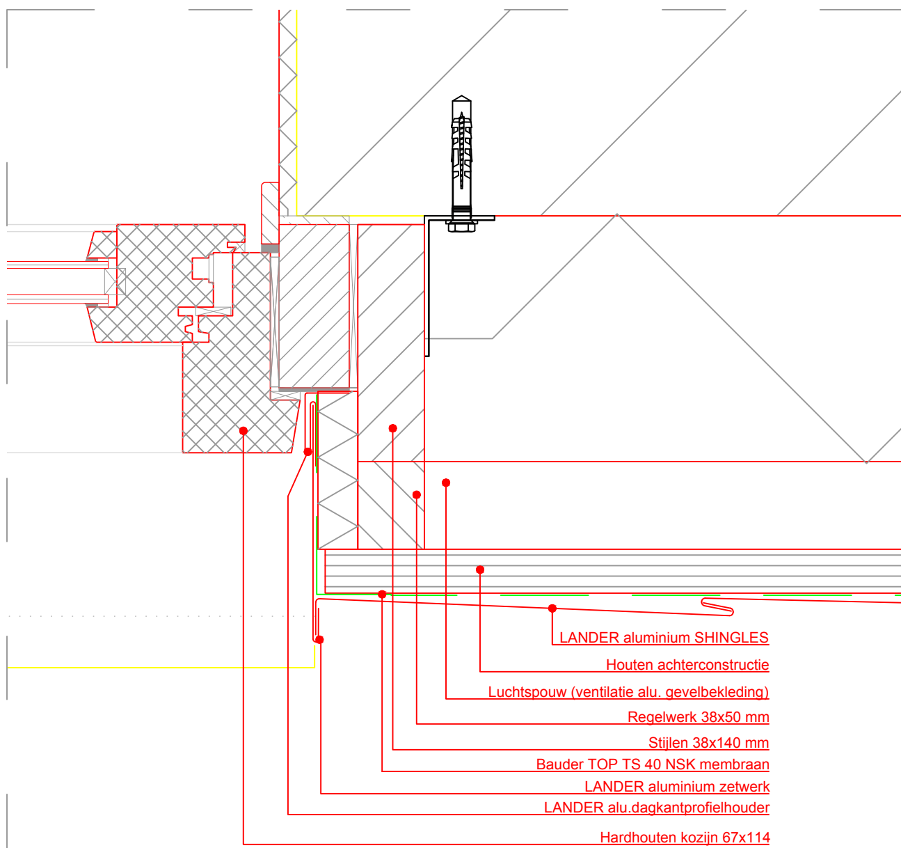
Aansluitdetail kozijnstijl H-03c
