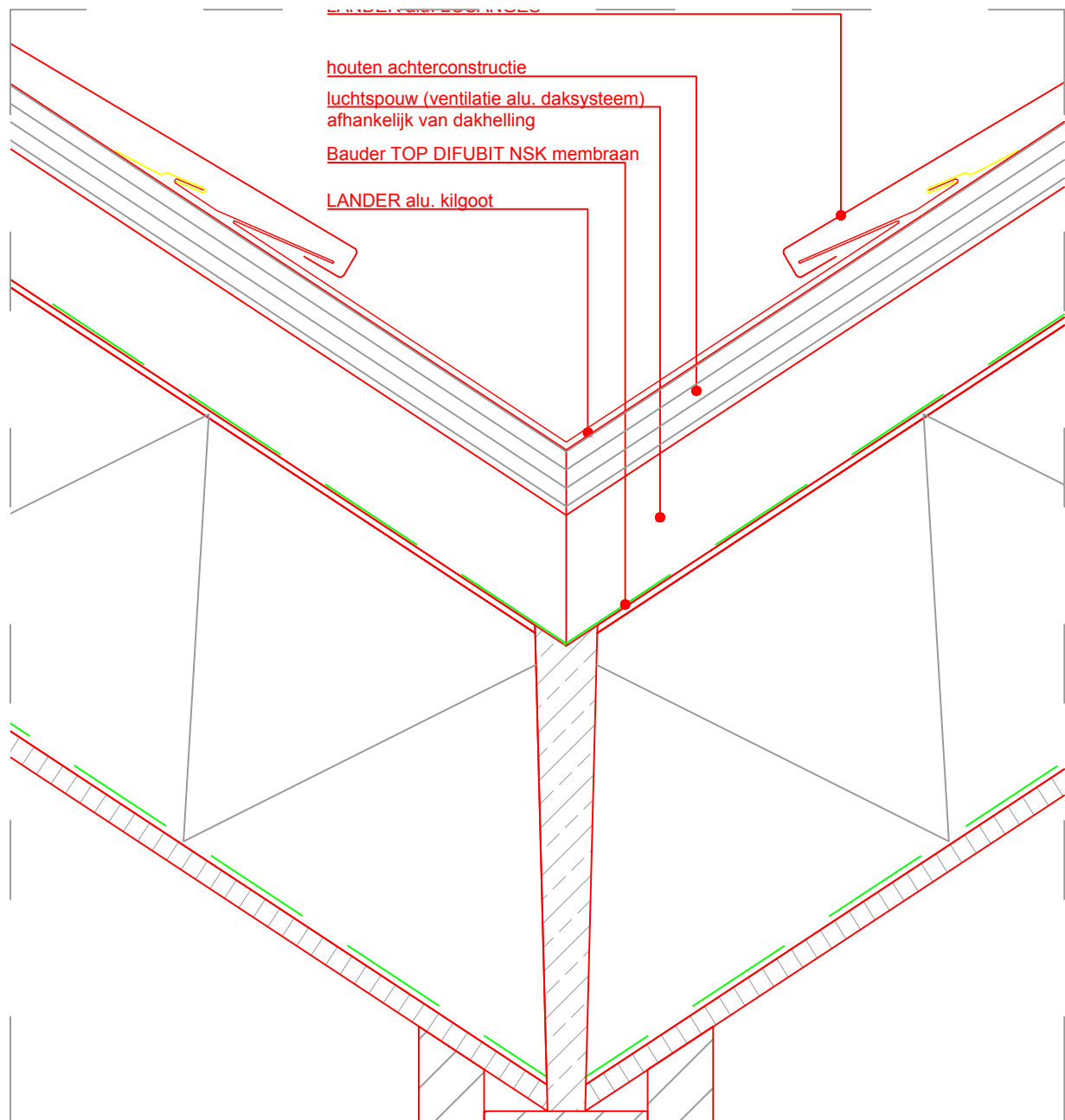
Kilkeperdetail H-02
