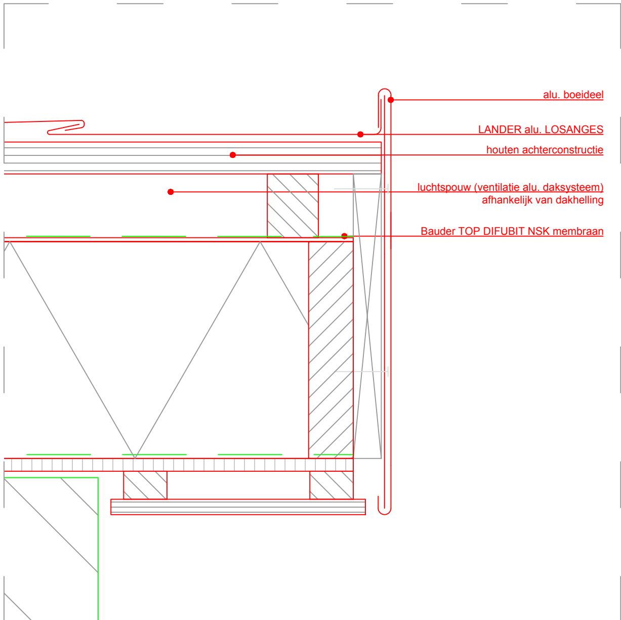
Topgeveldetail H-03
