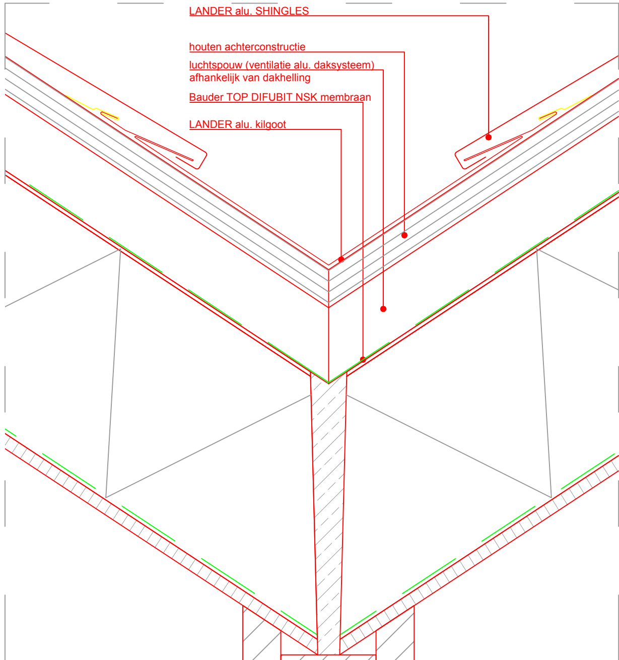
Kilkeperdetail H-02
