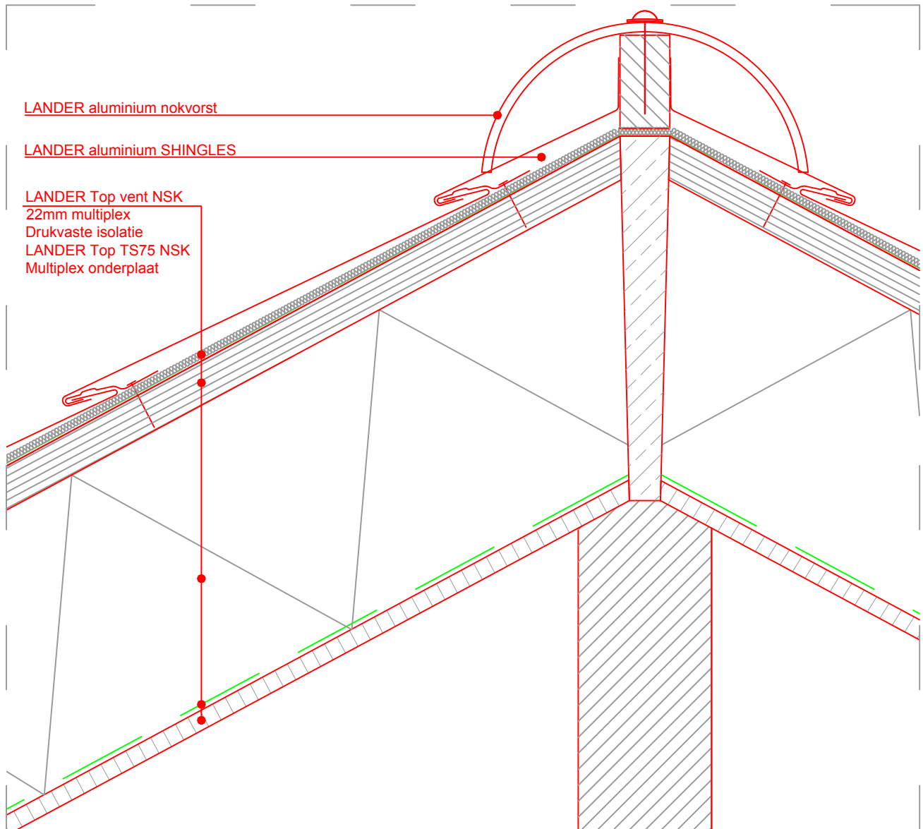
Hoekkeperdetail H-01m
