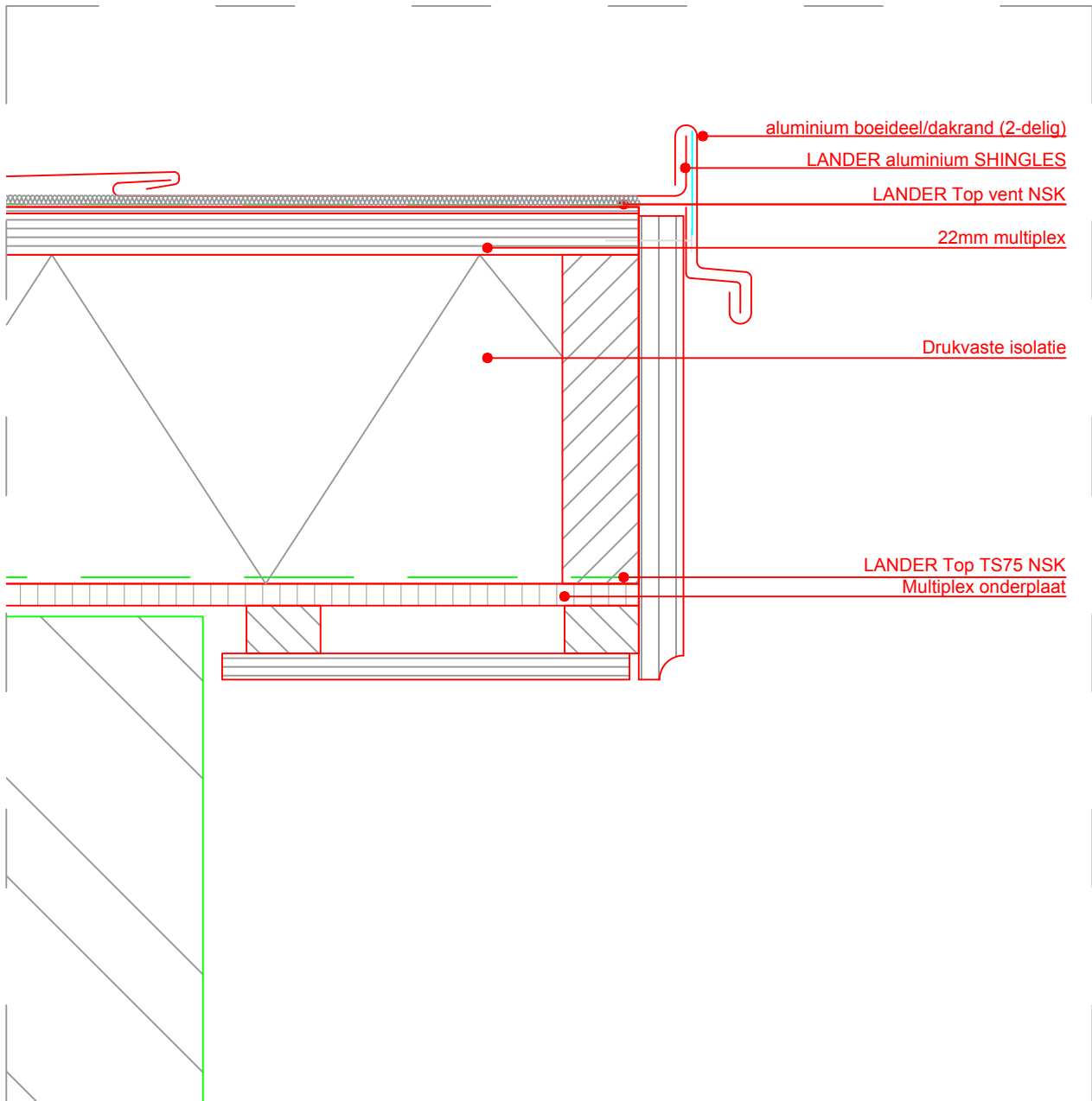
Topgeveldetail H-03m(a)
