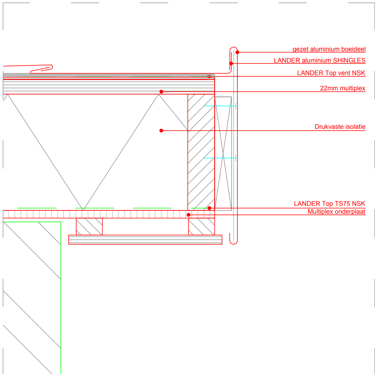
Topgeveldetail H-03m
