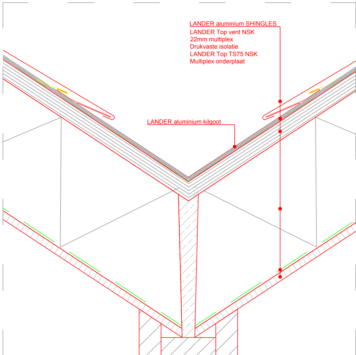
Kilkeperdetail H-02
