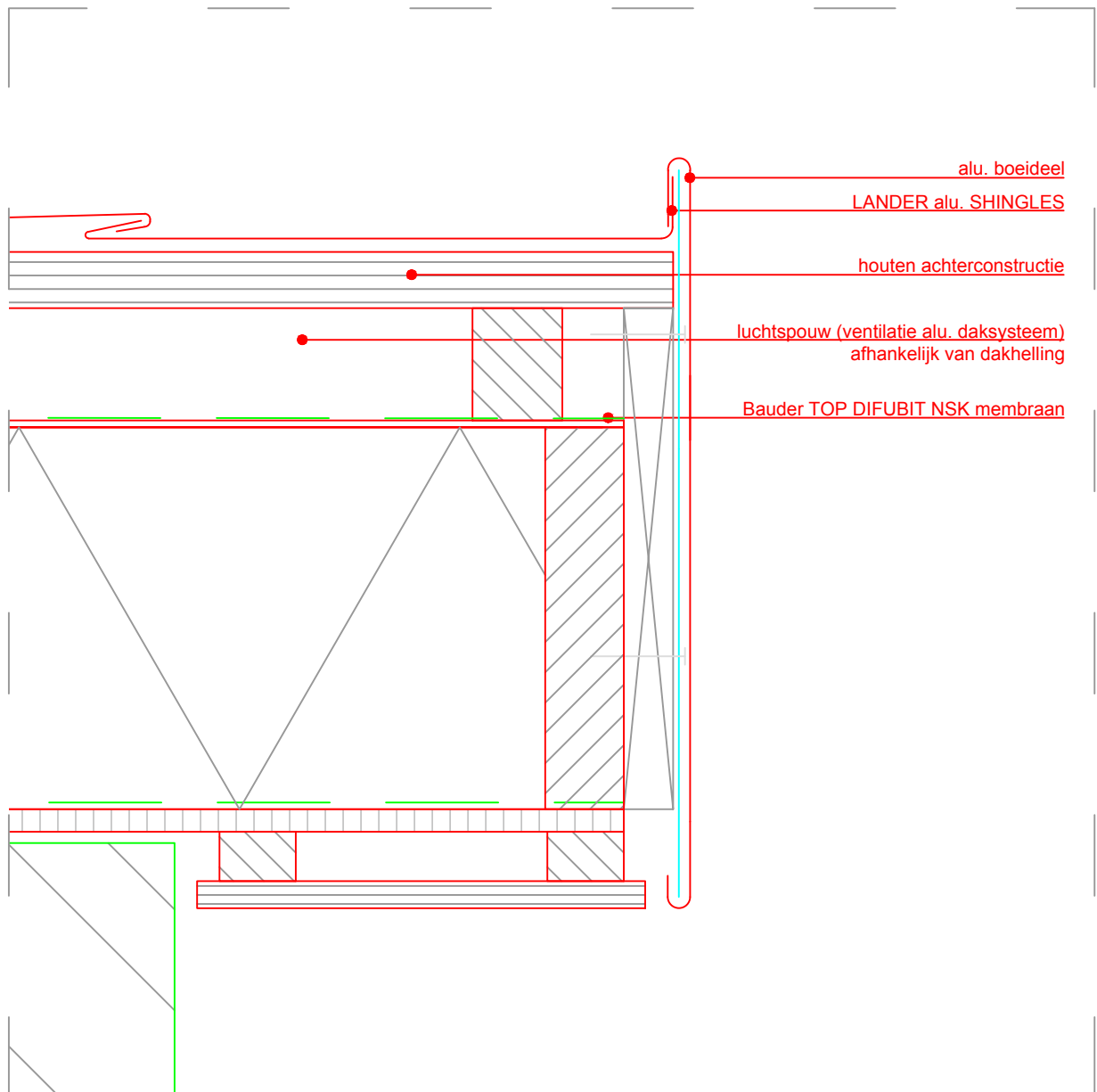
Topgeveldetail H-03
