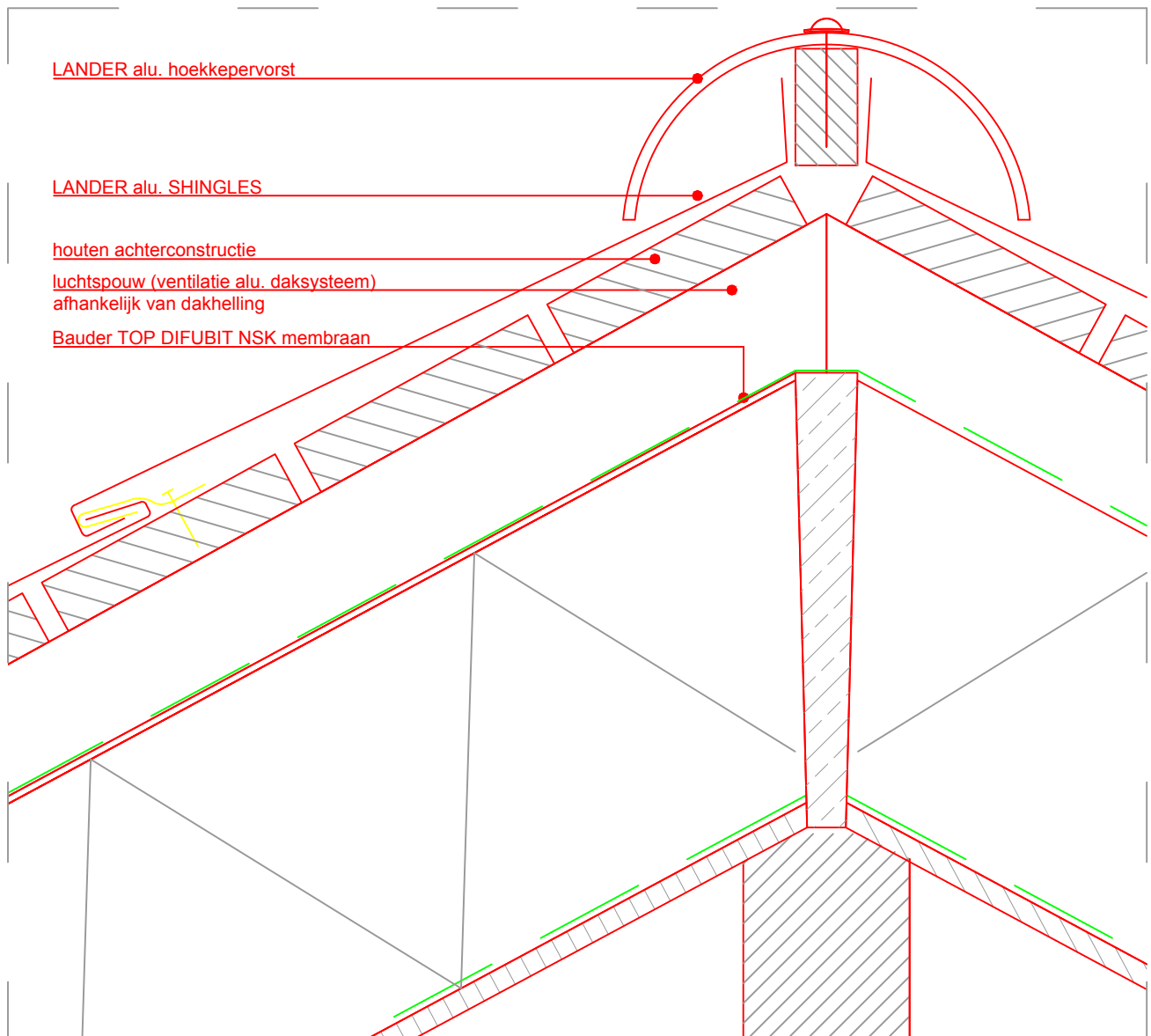
Hoekkeperdetail H-01
